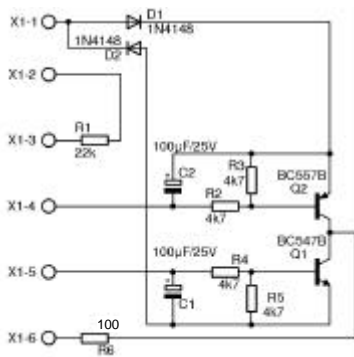
Fig. 1: Schaltplan
